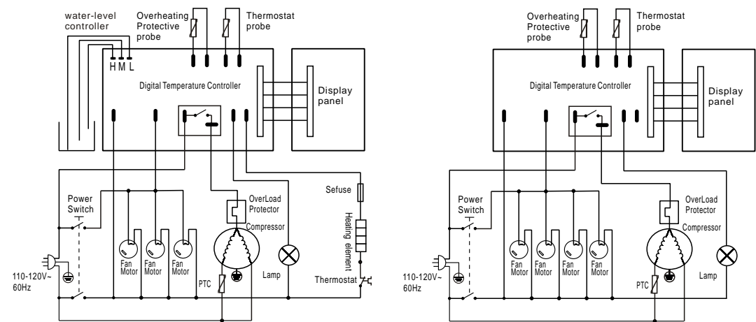
RTS-390LS_/RTS-390LS
